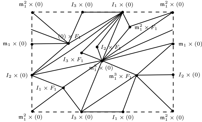
Fig 2.18: Torus embedding of \mathbb{A}\mathbb{G}(R_1 \times F_1) with n_1 = 4 , I_i m_1^i \neq (0) \forall i , I_1 m_1^2 = (0) , I_i m_1^2 \neq (0) \forall i \neq 1 and I_1 I_2 = I_1 I_3 = (0)
